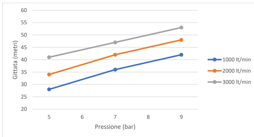
Grafico gittata FI-ABA BZ
